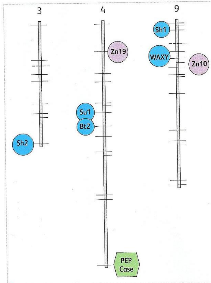
b Carte génétique simplifiée des chromosomes 3, 4 et 9 du maïs.
